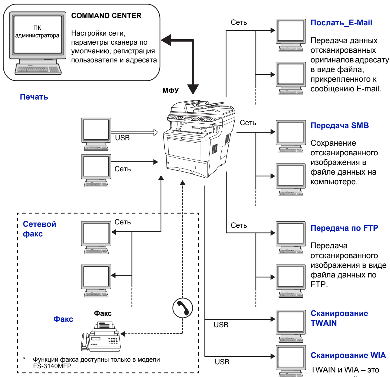
Подключение сканера к компьютерной сети с помощью сетевого кабеля (100BASE-TX или 10BASE-T)
